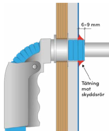
4.6.3h Tätning mot skyddsror vid plastmatta som tät- och ytskikt.
