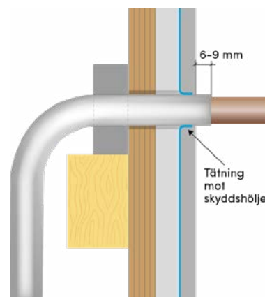
4.6.3f Tätning mot plathölje vid keramiskt ytskikt.
