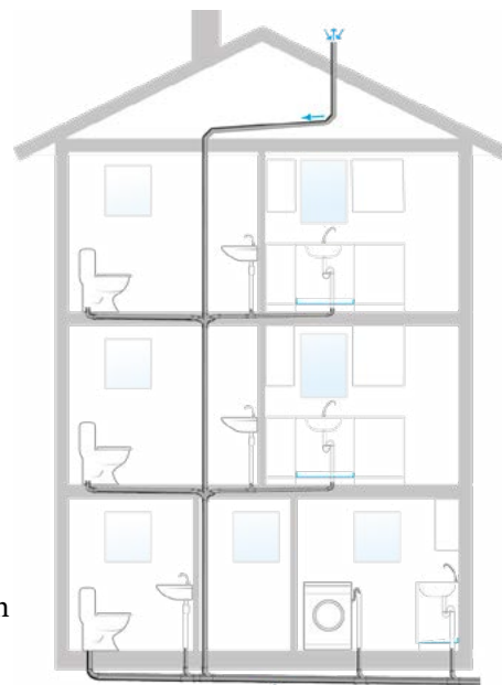
4.4.4a Luftning av flerbostadshus.
