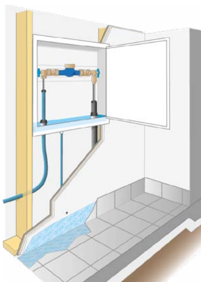
4.2.4a Vattenmätarskåp.
