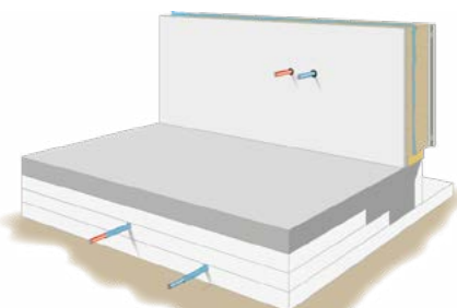
4.1.8c Exempel på rörförläggning av kall- och varmvatten i isolering vid platta på mark.
