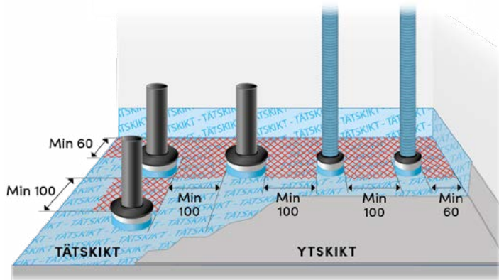
U4.6.1a Exempel på rör genomföringshylsa.
