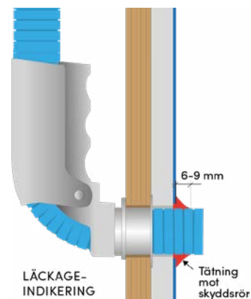
4.6.3k Tätning mot läckageindikering vid plastmatta som tät- och ytskikt.
