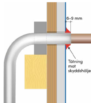
4.6.3i Tätning mot plathölje vid plastmatta som tät- och ytskikt.
