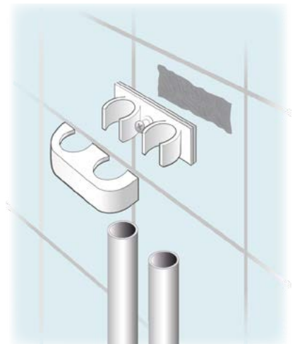
4.7.3a Infästning med lim.
