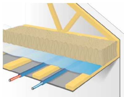
4.1.8b Exempel på rörförläggning på "varma sidan" i vindsbjälklag.
