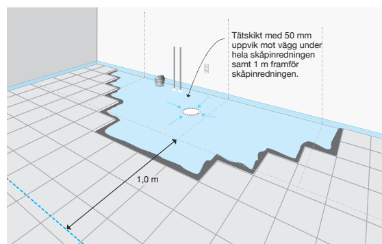
Vattentätt skikt under klinkergolv i kök.
