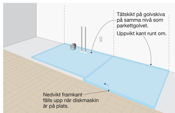
Prefabricerat tättskikt.
